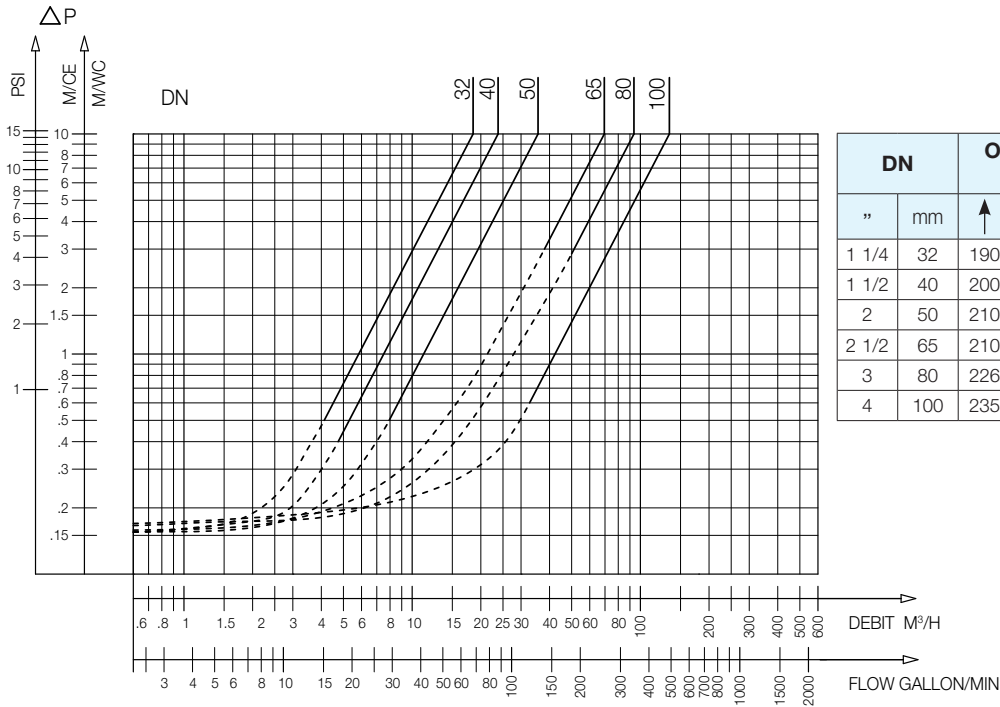
802L - Headloss chart
